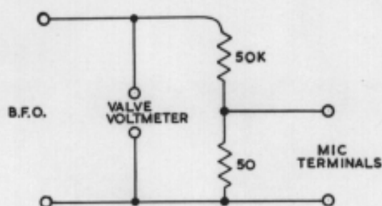
Fig. 9 Attenuator Pad
